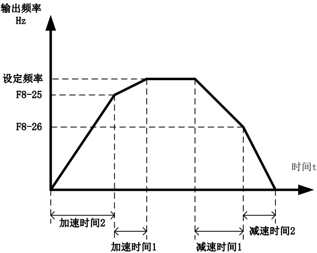
图 7-19 加减速时间切换示意图
