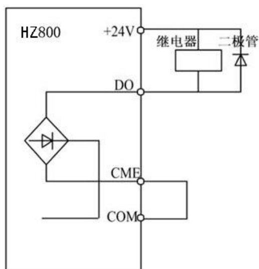
图 4-3 数字输出端子接线示意图
