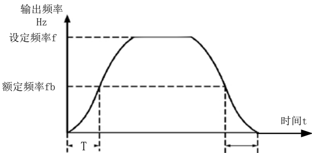
图 7-12 S 曲线加减速 B 示意图
