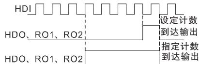
图6-18 设定计数值和指定计数值示意图
