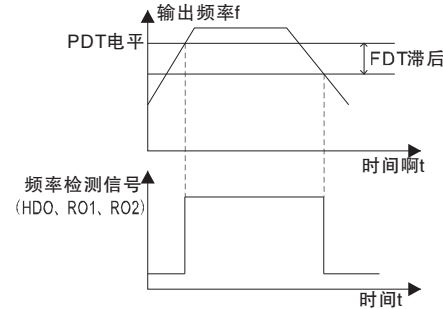
图6-19 FDT电平示意图
