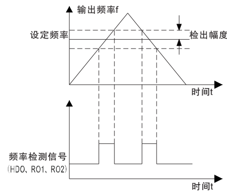
图6-20 频率到达检出幅值示意图
