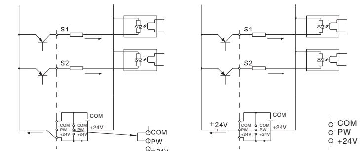
图4-15 共集电极模式
