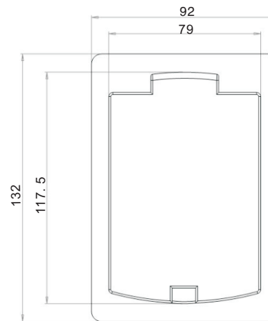
图A-7 外引键盘安装尺寸
