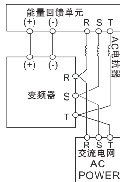
图4-18 能量回馈单元连接图
