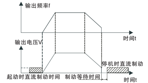
图6-3 直流制动示意图
