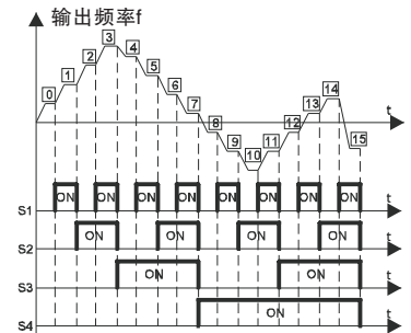
图6-25 多段速度运行逻辑图
