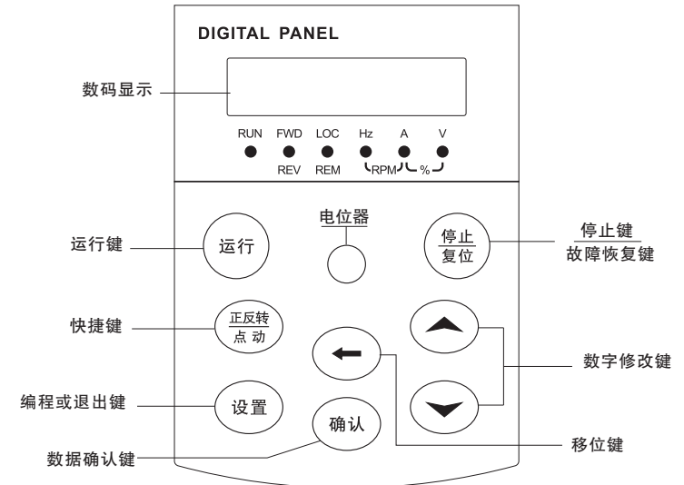
图5-1 键盘示意图
