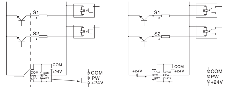
图4-14 共发射极模式
