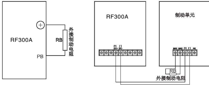
图 B-1 制动电阻的安装
