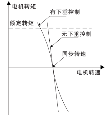
图6-21 下垂控制电机特性示意图
