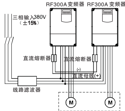
图4-19 共直流母线的连接
