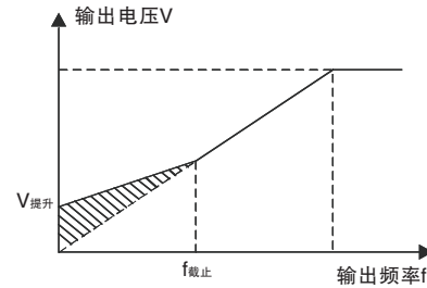
图6-7 手动转矩提升示意图
