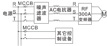
图4-16: 主回路电源侧连接图
