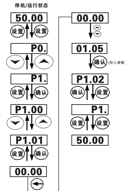
图5-2 三级菜单操作流程图
