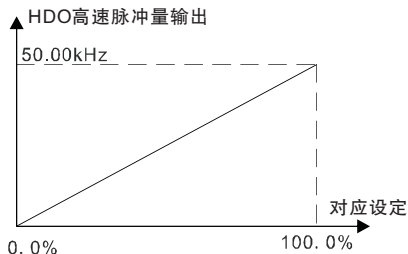
图6-15 给定量与高速脉冲输出对应关系
