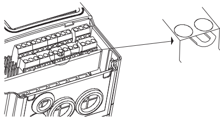
图4-13 U型短接片
