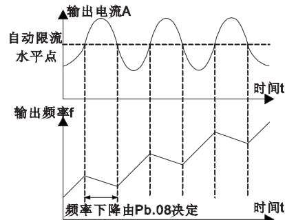
图6-29 限流保护功能示意图
