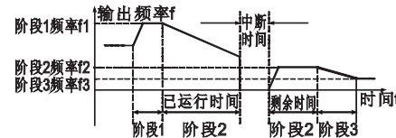
图6-26 简易PLC启动方式1
