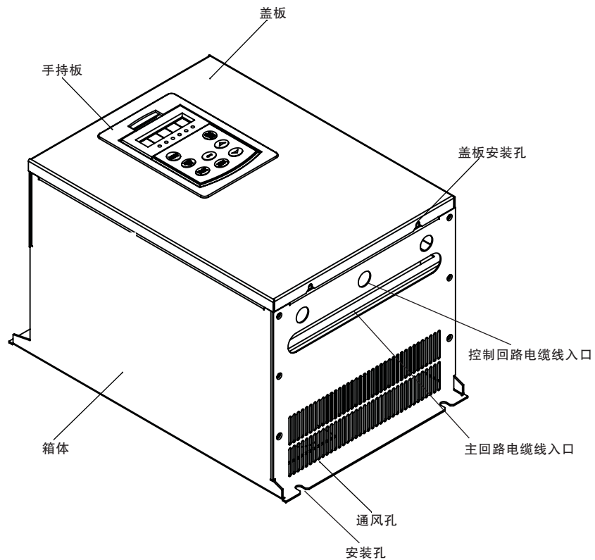
图1-2 变频器各部件名称
