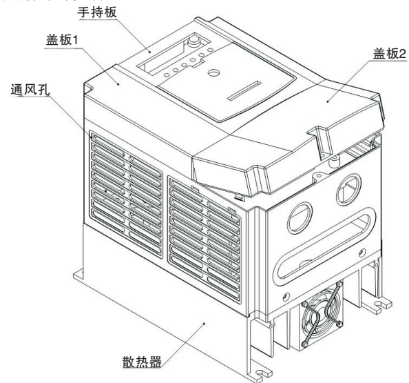
图A-8 塑胶盖板的安装与拆卸示意图
