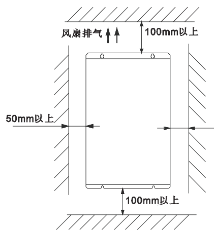
图 A-5 安装的间隔距离
