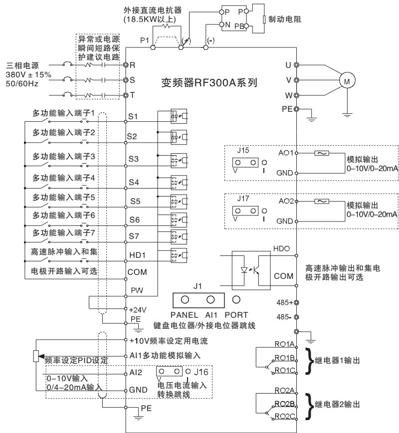
图4-12 标准接线图
