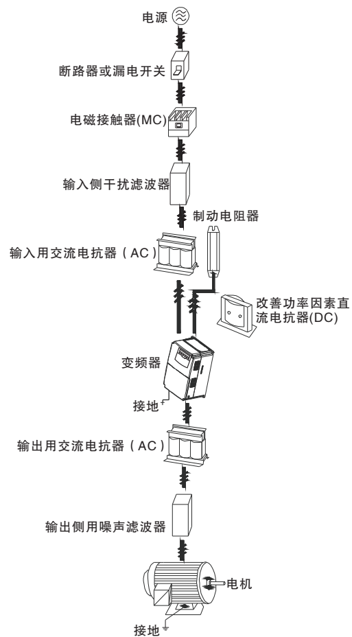
图4-1 外围设备的连接图
